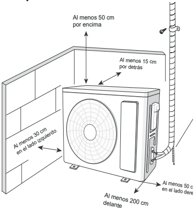
Configuración de las conexiones frigoríficas
