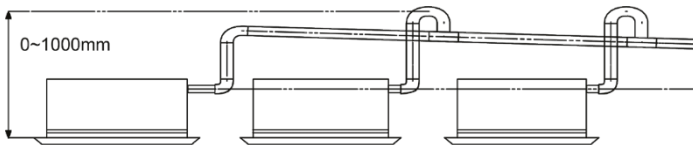
Condensaatleidingen die samenkomen in een T-stuk
