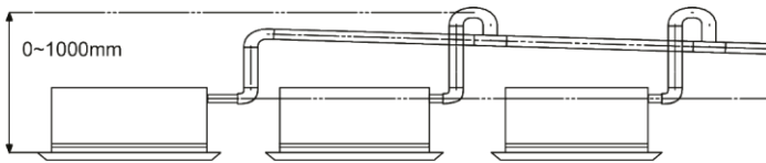
Tubos de condensación convergentes en una T
